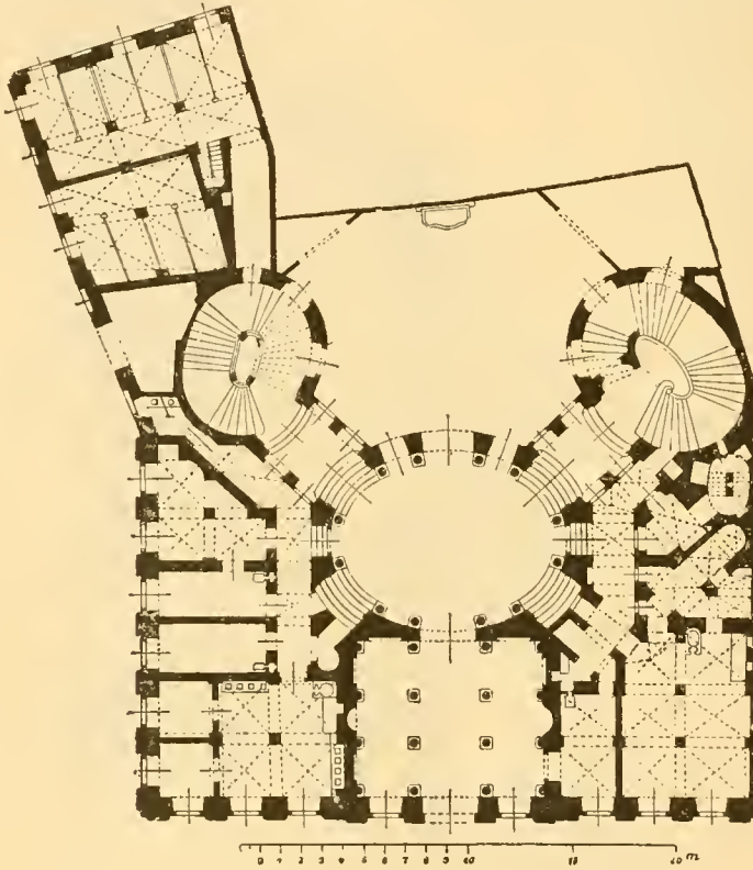
Fig. 143. Palais Schönburg zu Dresden. Grundriss des Erdgeschosses.
